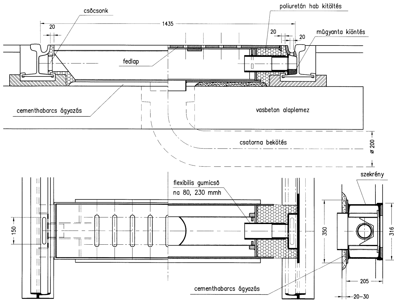
87. ábra. Víztelenítő szekrény RAFS rendszerű vágányhoz
