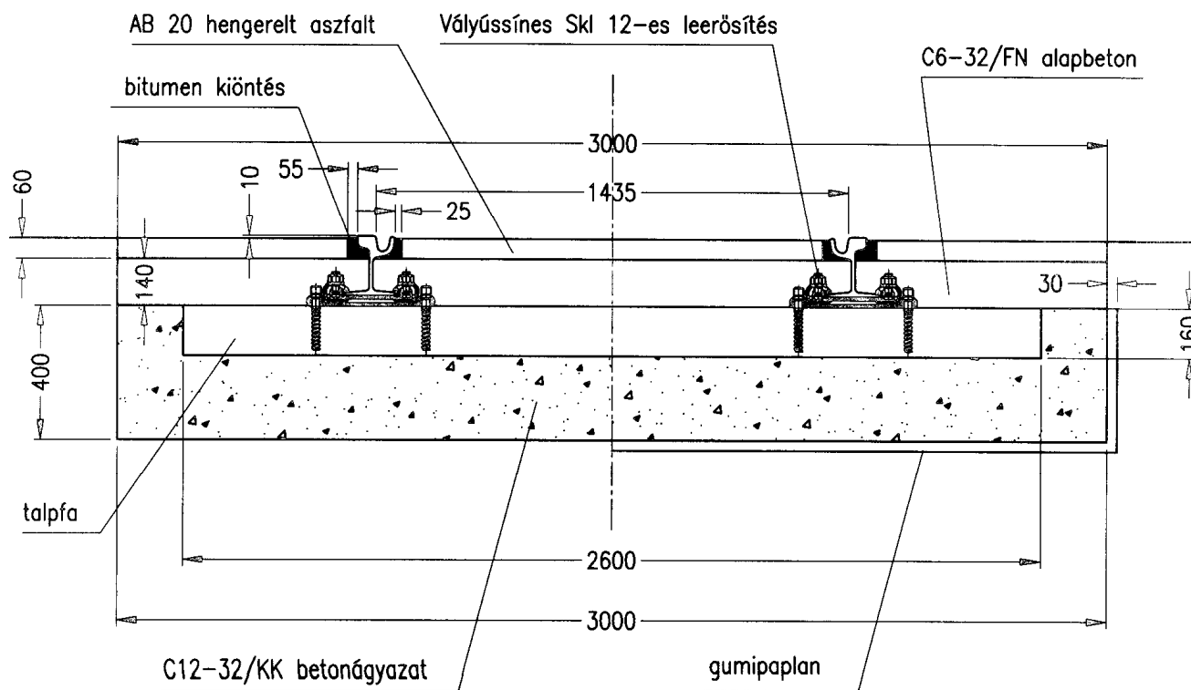
89. ábra. Vályússínes, bebetonozott talpfás vágány
